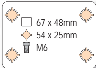
63mm swivel
